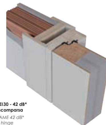
TELAIO EI30 con cerniera a scomparsa e/o a bandella EI30 FRAME with flap concealed hinge
